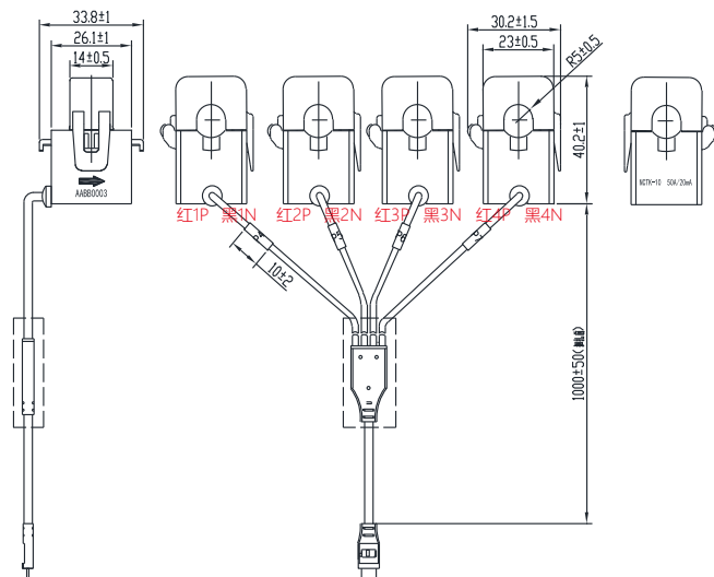
NTCK-10(50A*4) (一拖四)
