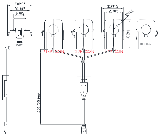
NTCK-10(50A*3) (一拖三)
