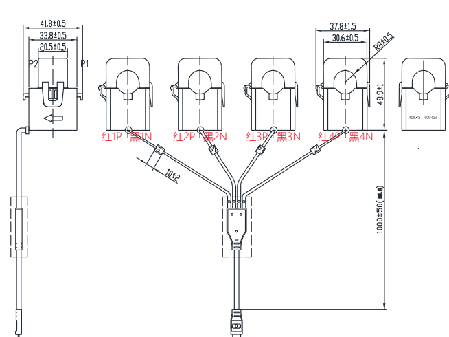
NTCK-10(100A*4) (一拖四)
